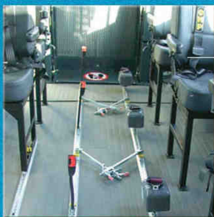
Ancoraggi carrozzina a pavimento con binari
